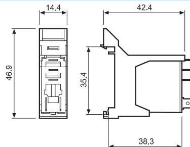
046.07 met relais
