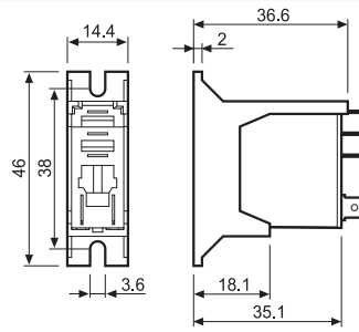
046.05 met relais
